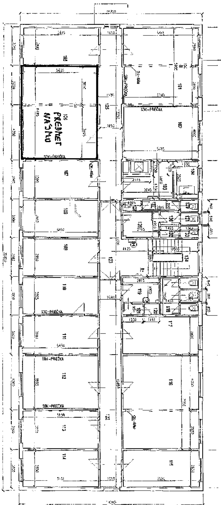
PÔDORYS POSCHODIA
